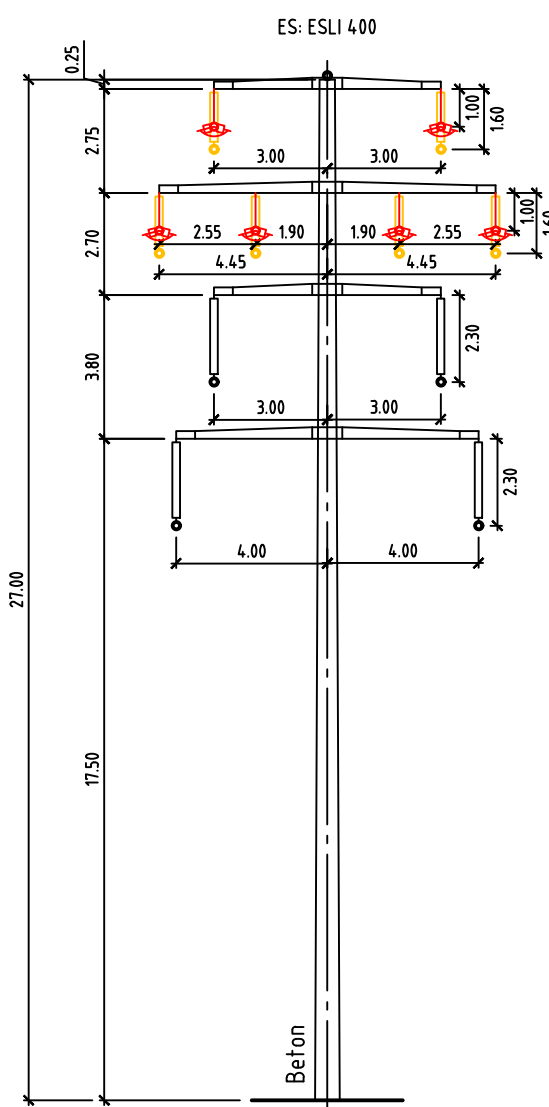
Mast 57 Tragmast einsteiig 110 kV / 132 kV Axpo / SBB
