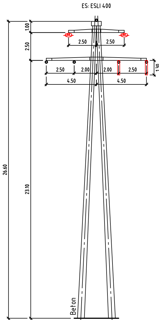
Mast 2 Abspannmast A-Bock quer 110 kV Axpo
