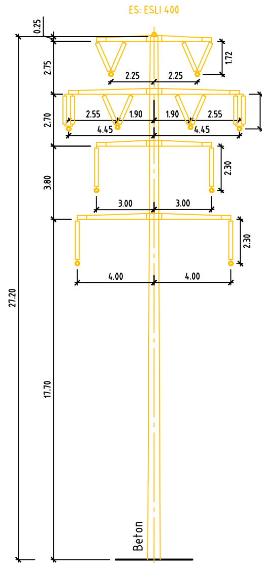
Mast 56 Tragmast einsteiig 110 kV / 132 kV Axpo / SBB
