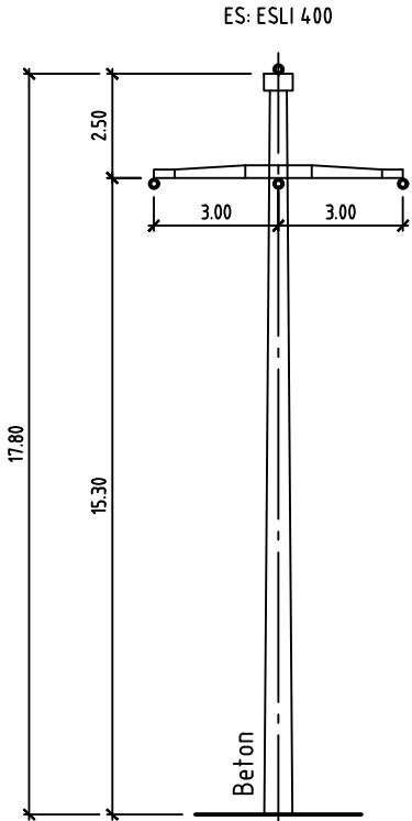
Mast 1B Endmast A-Bock längs 110 kV Axpo
