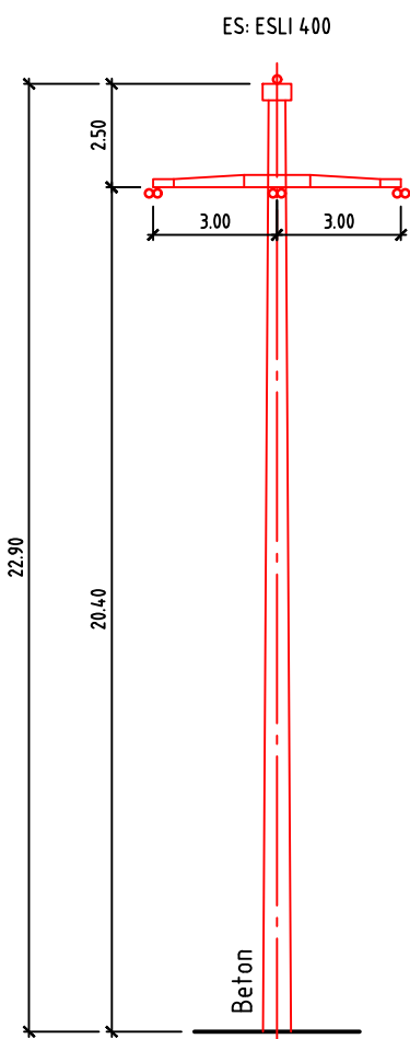
Mast 55A, 56A Endmast einsteiig 110 kV Axpo
