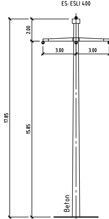
Mast 61B Endmast A-Bock längs 110 kV Axpo
