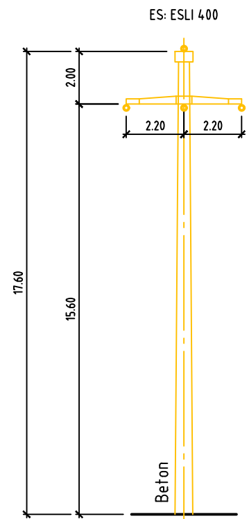
Mast 61A Endmast A-Bock längs 110 kV Axpo
