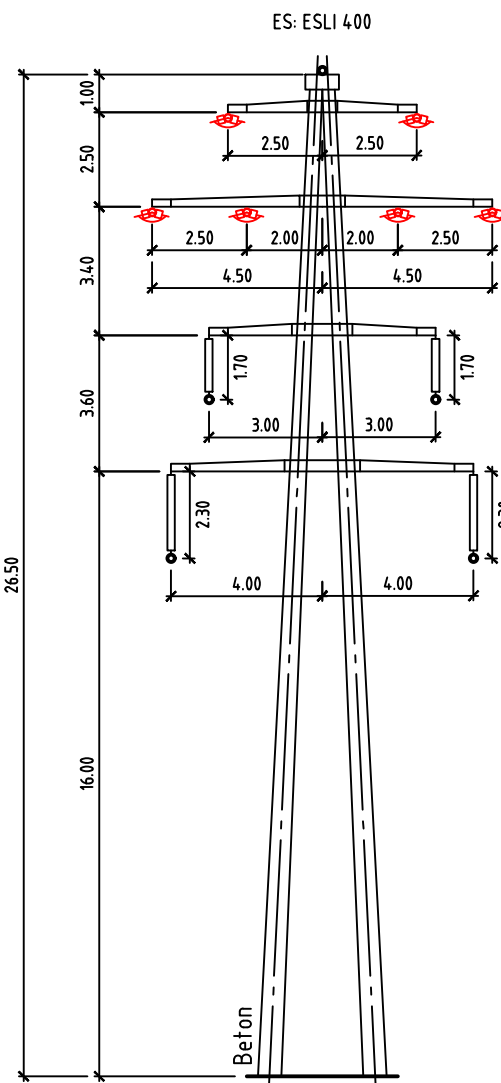
Mast 60 Abspannmast A-Bock quer 110 kV / 132 kV Axpo / SBB
