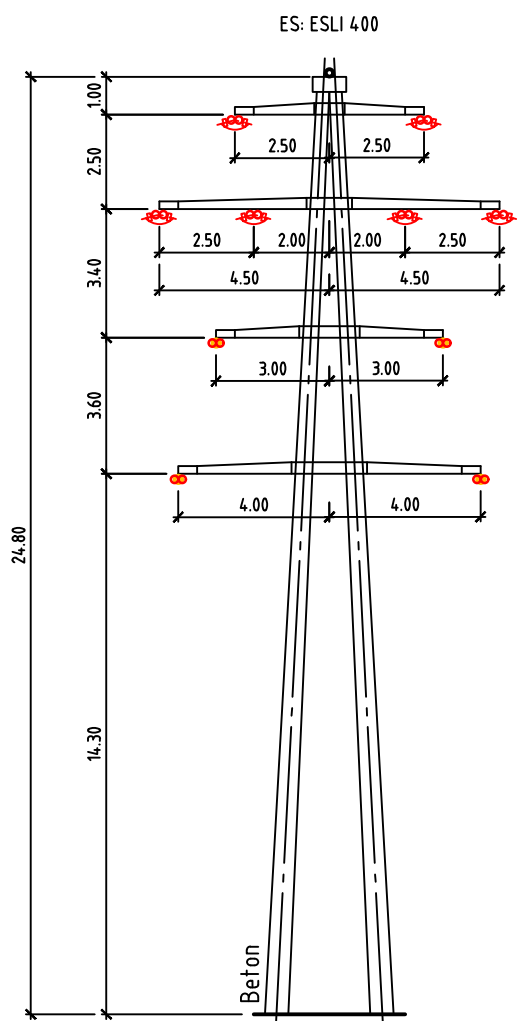
Mast 55 Abspannmast A-Bock quer 110 kV / 132 kV Axpo / SBB
