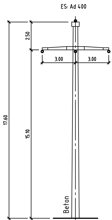
Mast 1A Endmast A-Bock längs 110 kV Axpo
