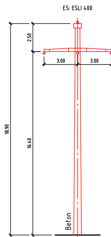
Mast 61AN Endmast einsteiig 110 kV Axpo
