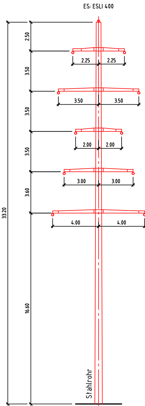
Mast 56N Abspannmast einsteiig 110 kV / 132 kV Axpo / SBB
