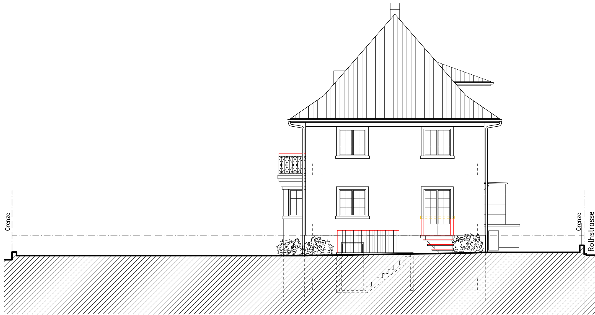
Fassade Süd-Ost
