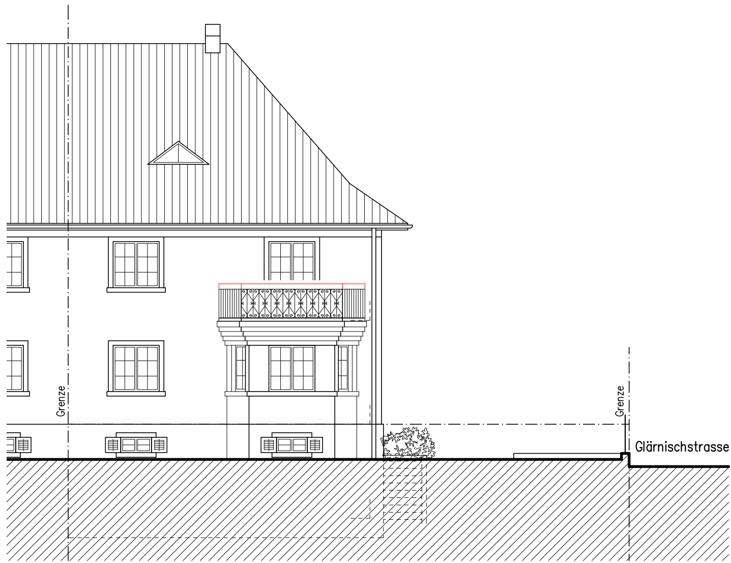
Fassade Süd-West
