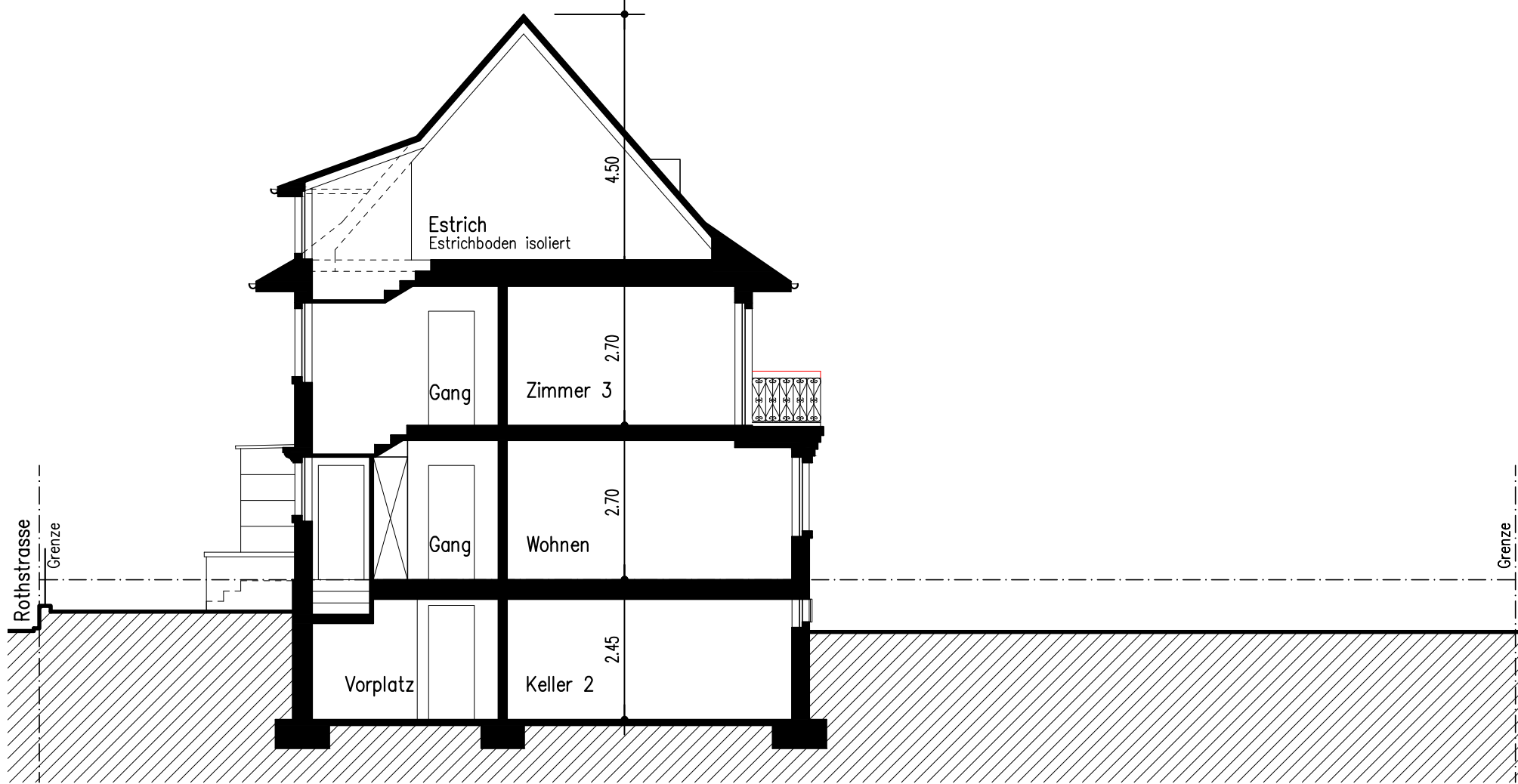
Schnitt A
