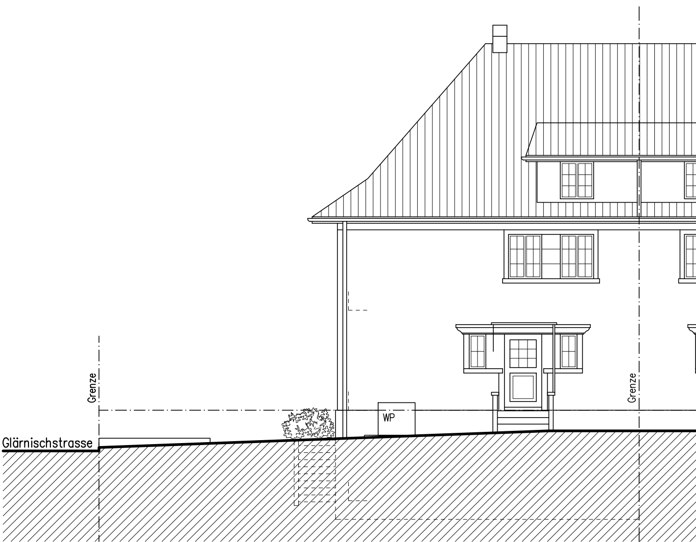
Fassade Nord-Ost
