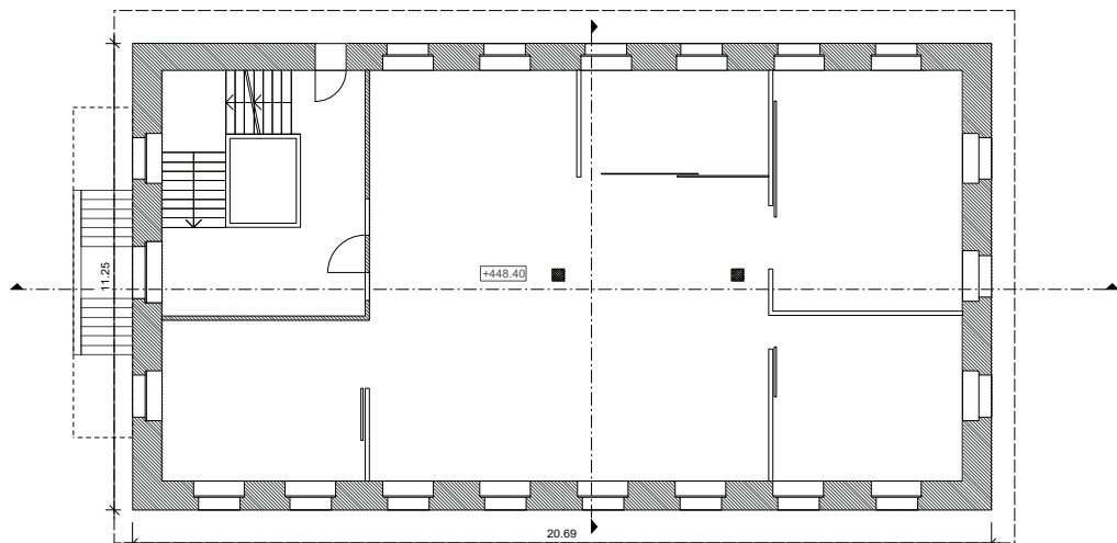
Grundriss Ebene 1
