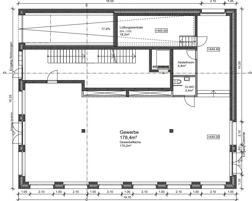
Grundriss Erdgeschoss
