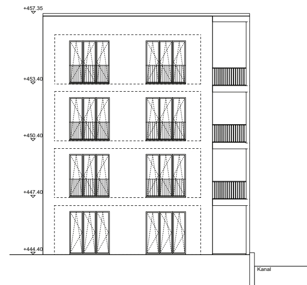
Ansicht Ost
