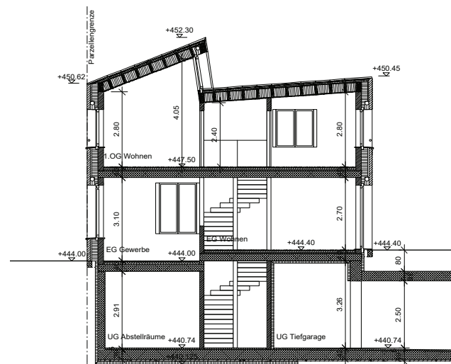
Querschnitt
