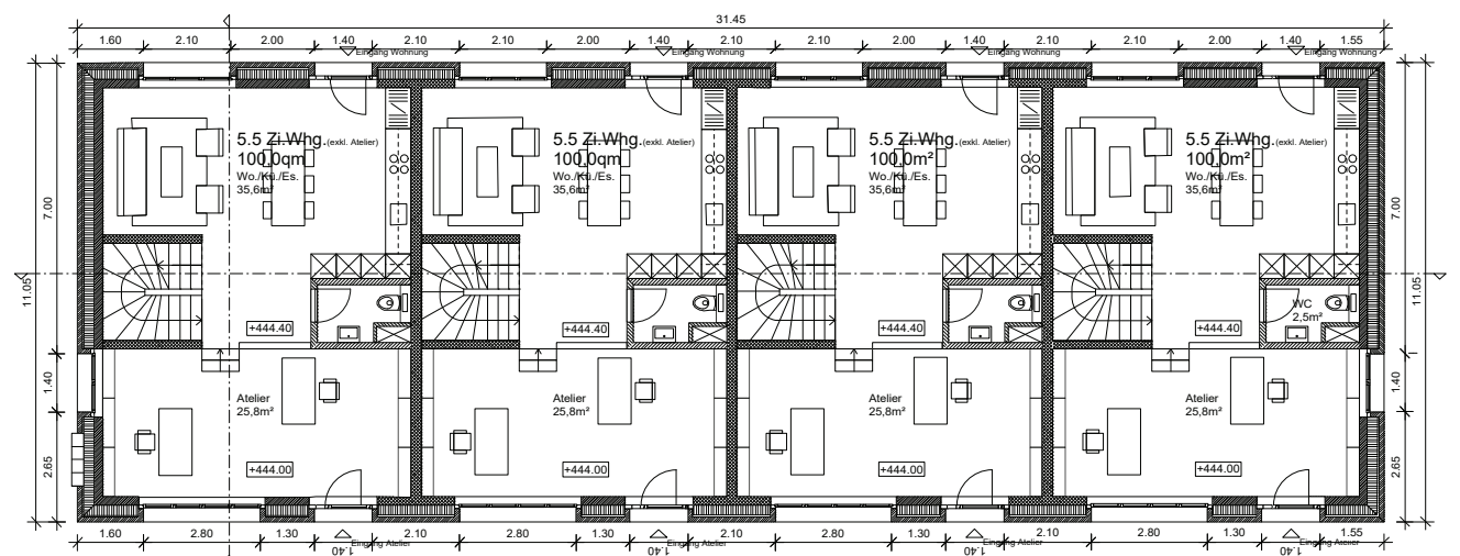
Grundriss Erdgeschoss
