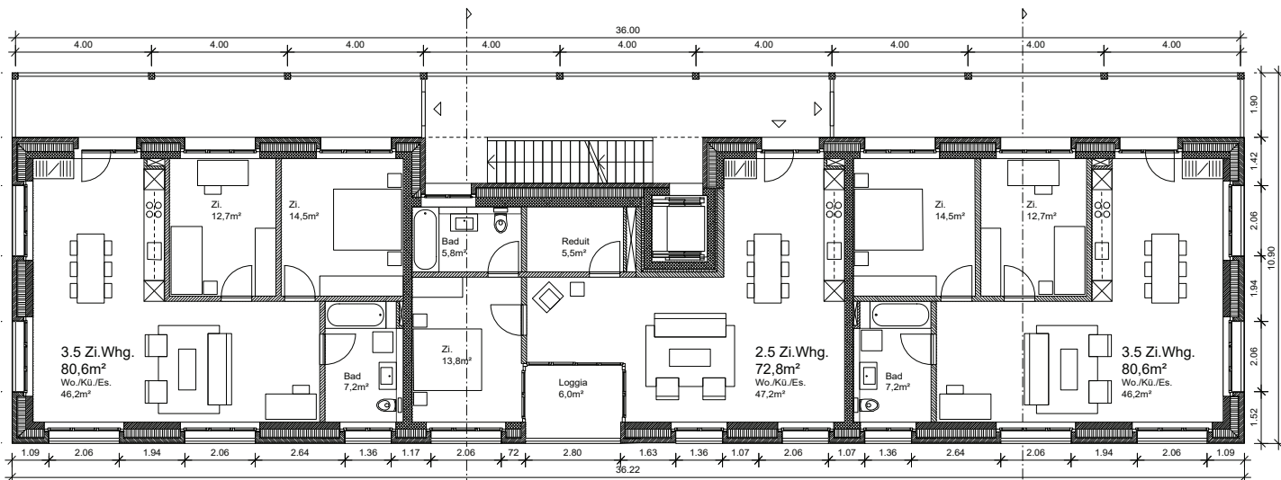
Grundriss 1.-3. Obergeschoss
