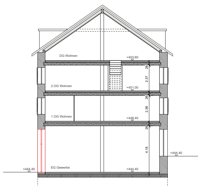
Querschnitt
