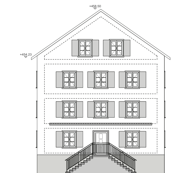
Ansicht Ost (Innenhof)
