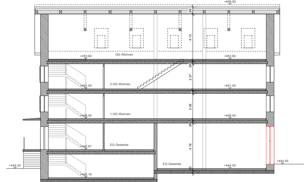
Längsschnitt
