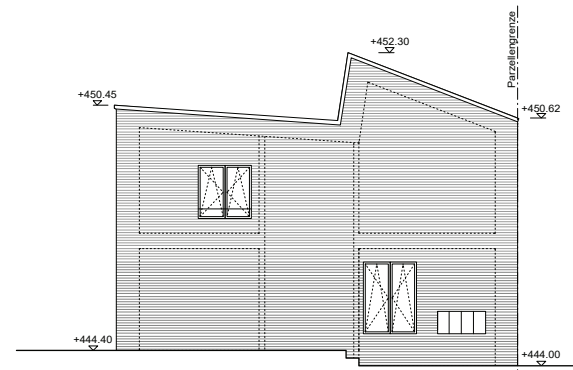
Ansicht West
