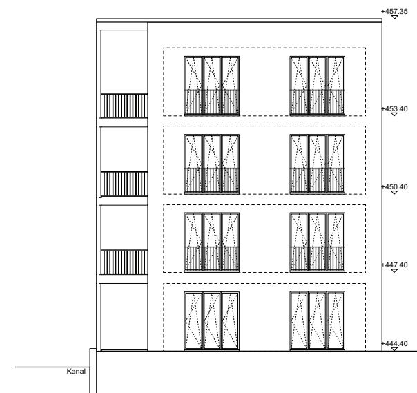
Ansicht West
