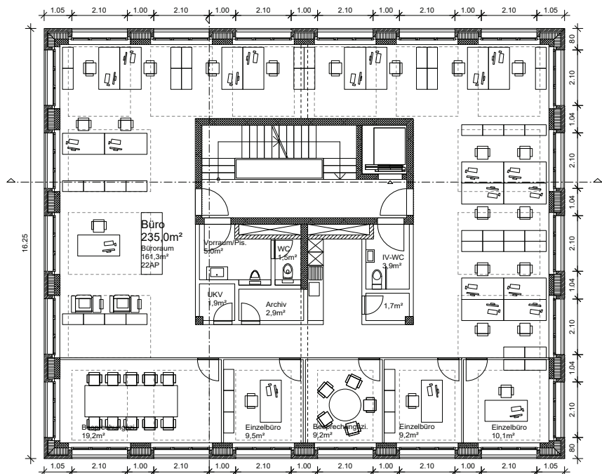
Grundriss 1. Obergeschoss
