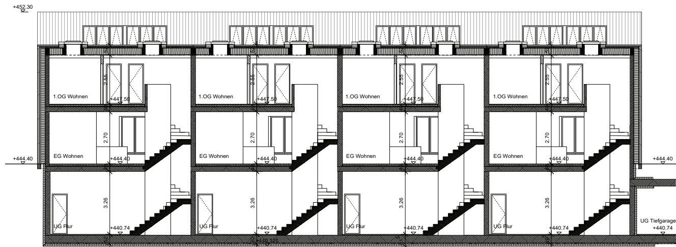
Längsschnitt
