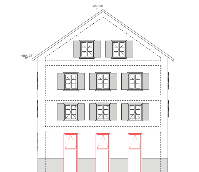
Ansicht West
