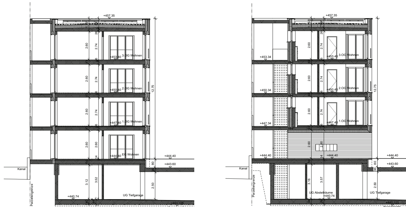
Schnitt Wohnung
