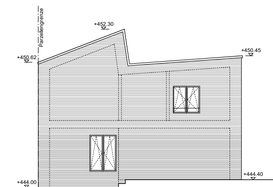
Ansicht Ost
