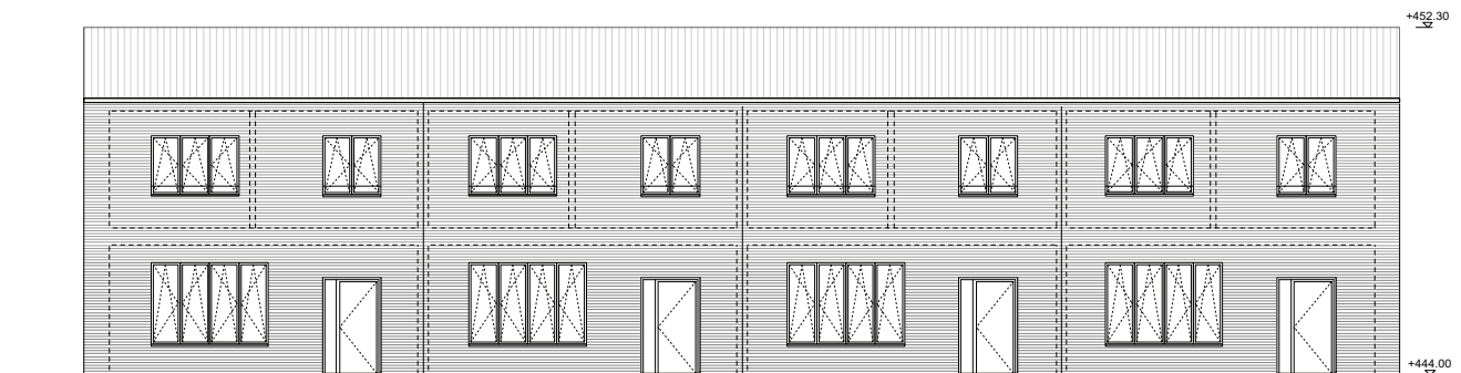
Ansicht Nord (Innenhof)
