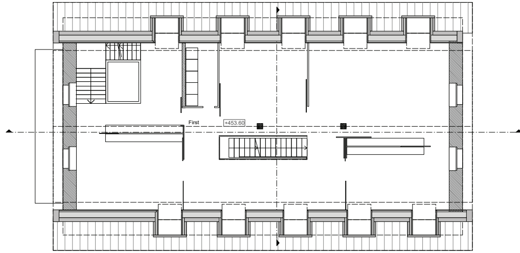
Grundriss Ebene 3
