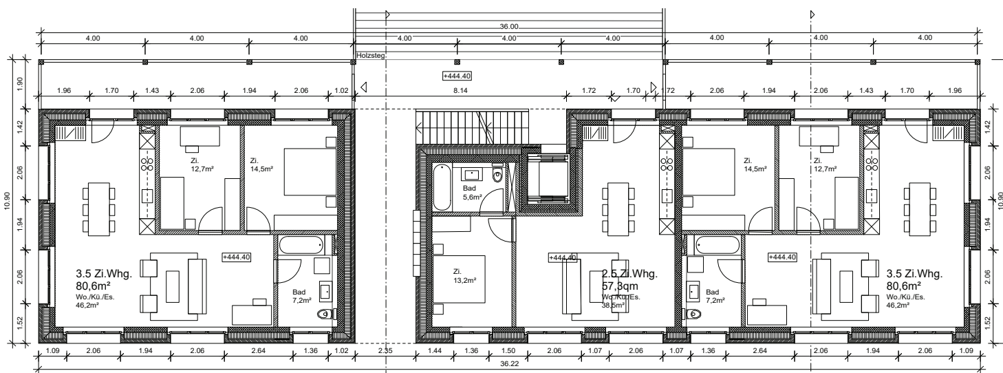
Grundriss Erdgeschoss
