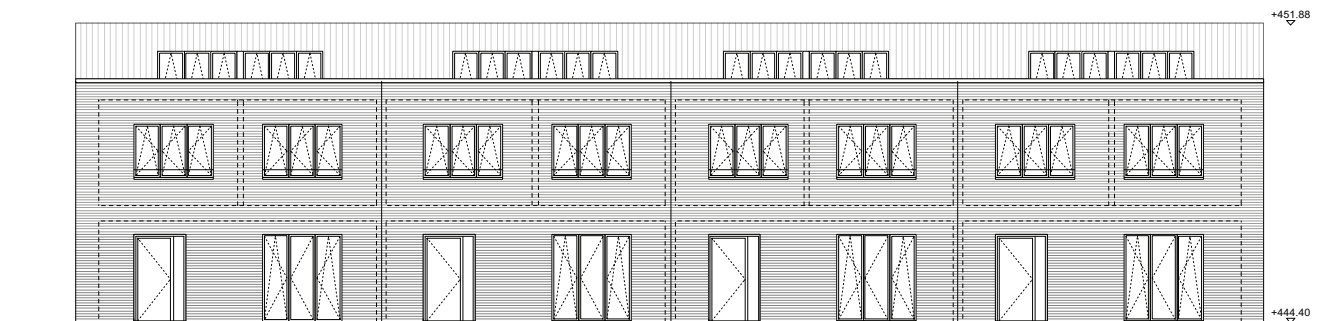
Ansicht Süd (Strasse)
