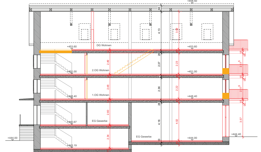
Längsschnitt
