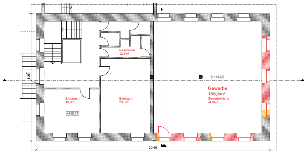
Grundriss Ebene 0
