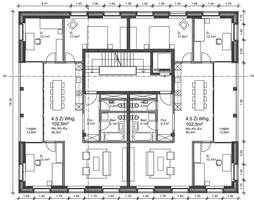
Grundriss 2.+3. Obergeschoss
