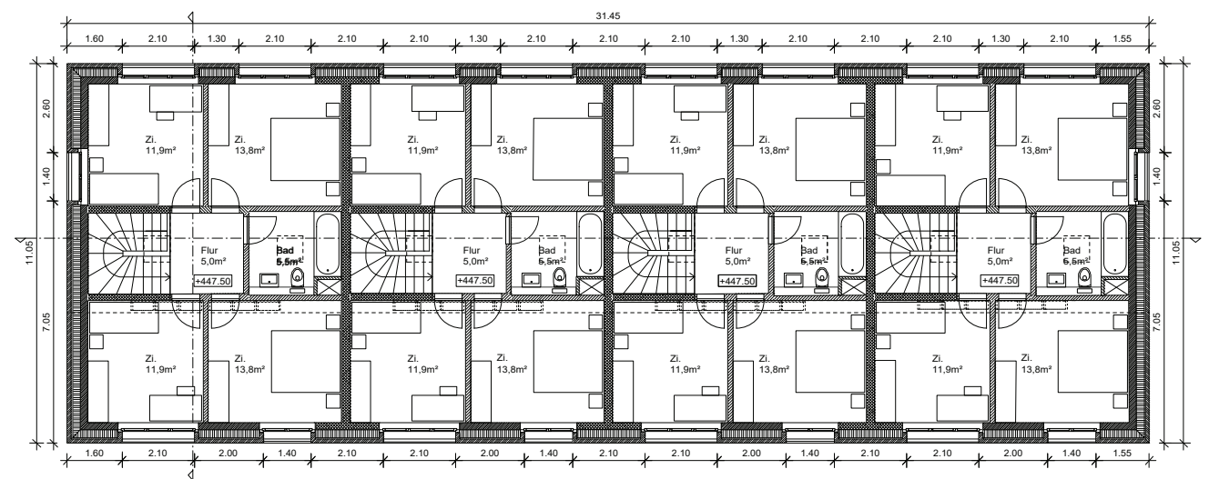
Grundriss 1.Obergeschoss
