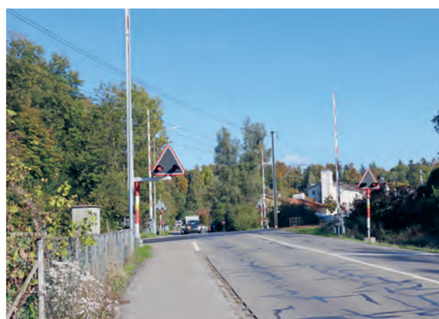
Abbildung 29: Bahnübergang Aathalstrasse.
