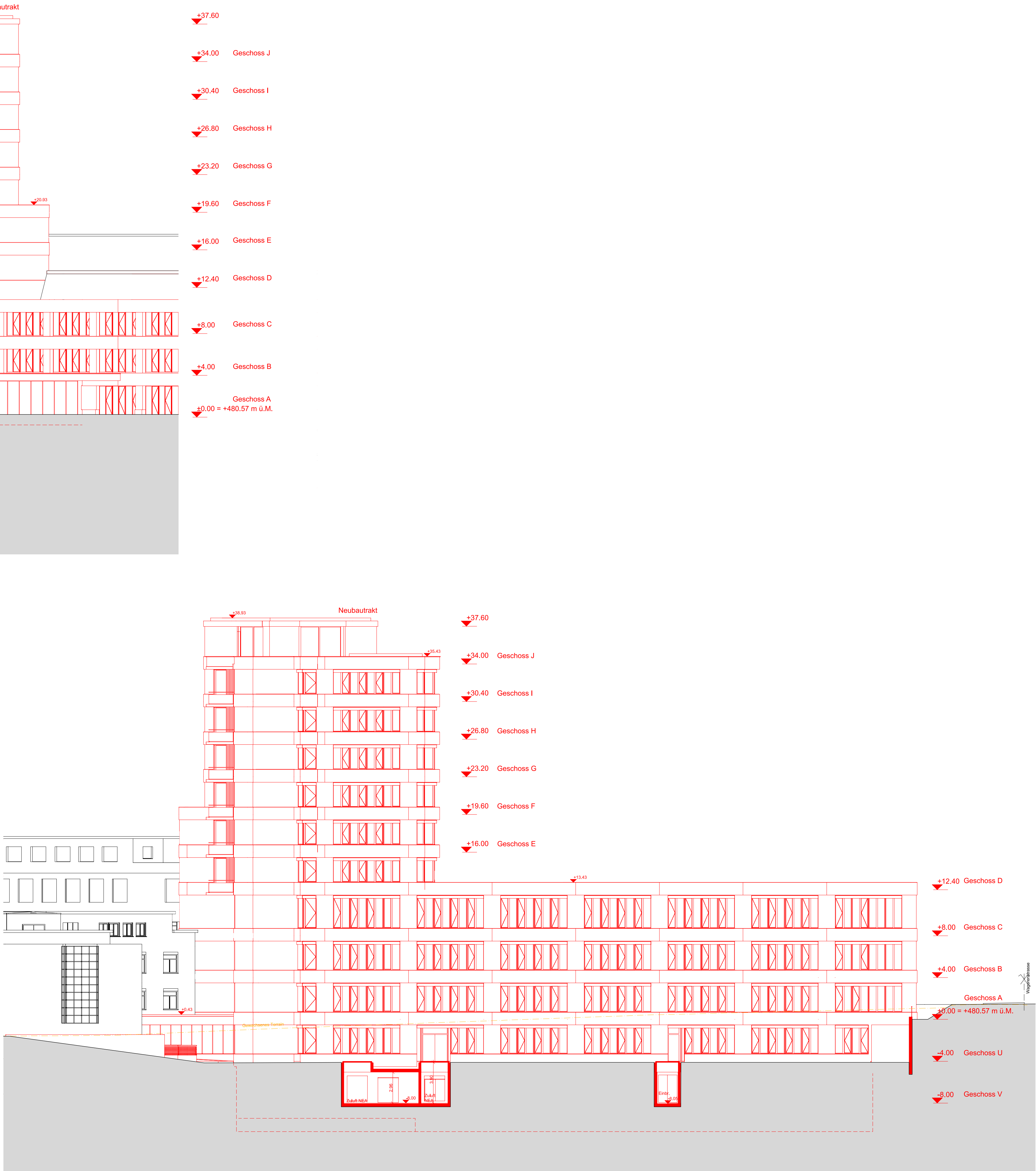
TO3 Westfassade
